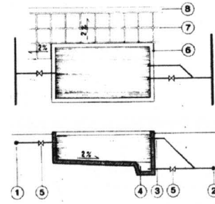
Schemat instalacji doprowadzających i odprowadzających wodę: 1. instalacja wodociągowa, 2. instalacja kanalizacyjna, 3. przewód, 4. osadnik, 5. zawór, 6. obrzeże basenu, 7. obójście wykonane z płyt kamiennych, 8. przykryta rynna odwadniająca obójście
