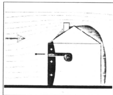
Na rys.: wiatr w sposób zasadniczy wpływa na skuteczność wentylacji grawitacyjnej
