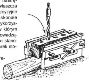
Presuwany się na trzpieniach klocek pozwala na centryczne wykonywanie otworów
