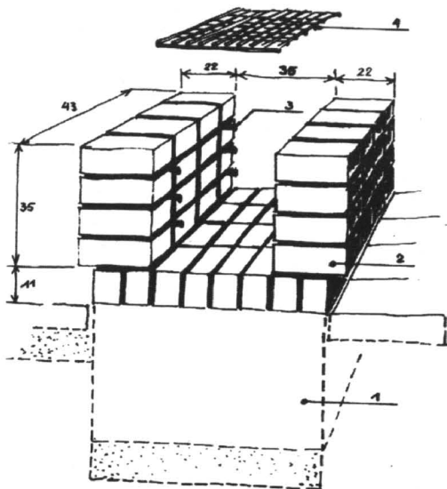
Rozeń ogrodowy wykonany z cegły klinkierowej (8x10x22 cm) 1. Fundament betonowy 2. Cegła klinkierowa 3. Pręty stalowe (Ø 8mm) 4. Ruszt
