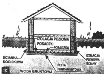
Budynek na terenie o wysokim poziomie wód gruntowych, sięgających powyżej dolnych części fundamentu
