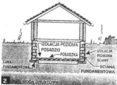
Budynek postawiony na terenie o niskim poziomie wód gruntowych, znajdującym się dużo poniżej dolnych części budynku
