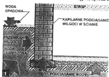
Część wody z opadów wsiąka w grunt, przedostaje się do wód gruntowych albo zatrzymuje się w warstwach wyższych
