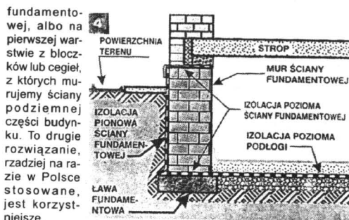
Izolację przeciwwilgociową układa się na zewnętrznej stronie ściany fundamentów
