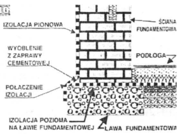
Izolacja pozioma na ławie fundamentowej
