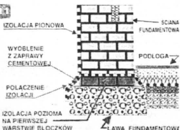
Izolacja pozioma na pierwszej warstwie bloczków
