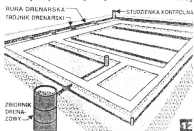
Drenaż posadzkowy wodę gromadzącą się pod posadzką ma odprowadzić do drenażu opaskowego
