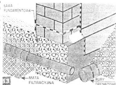
Aby odprowadzić wodę z systemu rur drenarskich trzeba przewidzieć przeprowadzenie ich przez mur
