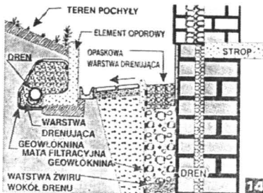
Drenaż wokół budynku posadowionego na sto-
