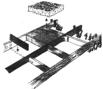
Rys. 1. Forma zespolona (szalowanie) do odlewu ozdobnych płyt cementowych
