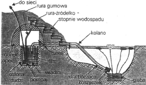
Tak wygląda kaskada „Od kuchni”
