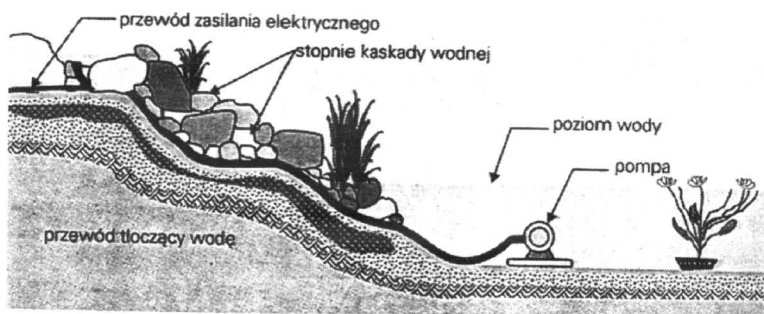
Kaskada wykorzystująca pompę zanurzeniową
