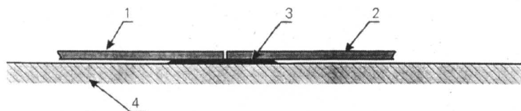
Mocowanie rolowanej wykładziny Vinigam do podłoża za pomocą taśmy dwustronnie klejącej: 1 - sąsiadujące ze sobą pasy wykładziny, 3 - taśma dwustronnie klejąca, 4 - podłoże
