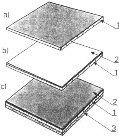
Budowa płytek podłogowych: a) płytka homogeniczna, b) płytka heterogeniczna Vinigam Rekord, c) płytka heterogeniczna Vinigam Rekord E. 1 - PCW, 2 - przezroczysta folia, 3 - spienione PCW
