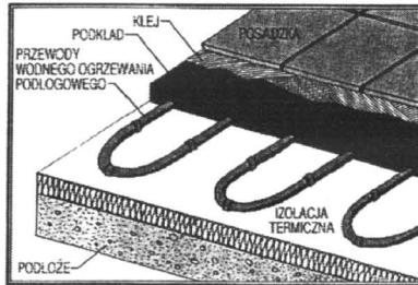
Schemat ogrzewanej podłogi z elektrycznymi lub wodnymi elementami grzejnymi
