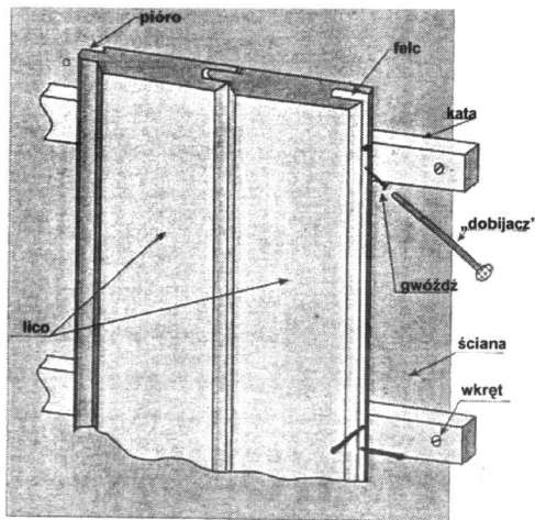
Prawidłowe przybijanie desek boazeryjnych do podkładu
