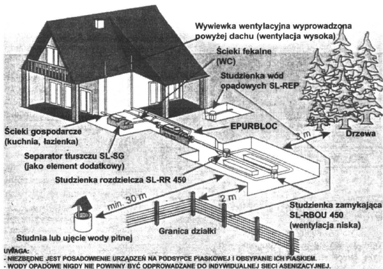
Rys. 1. Elementy niezbędne do zbudowania przydomowej oczyszczalni
