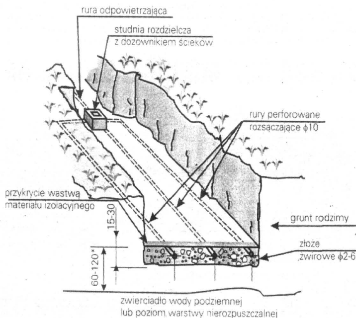
Rys. 2. Widok pola drenazowego
