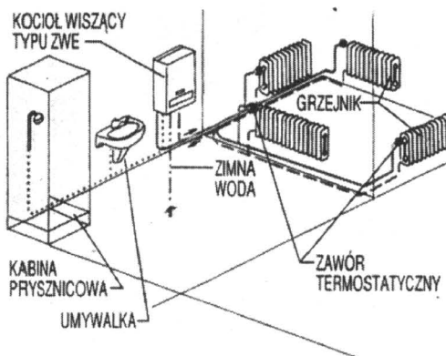
Rys. 4. Schemat instalacji zasilanej tylko kotłem dwufunkcyjnym
