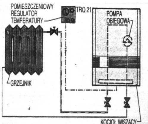
Rys. 5. Schemat instalacji c.o. z wiszącym kotłem jednofunkcyjnym
