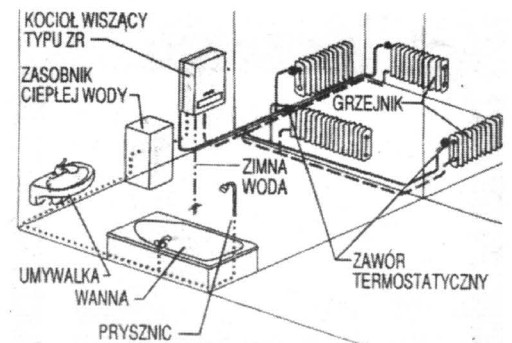
Rys. 3. Schemat instalacji zasilanej kotłem dwufunkcyjnym z zasobnikiem ciepłej wody
