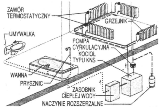
Rys. 2. Schemat instalacji zasilanej kotłem stacjonarnym z zasobnikiem ciepłej wody
