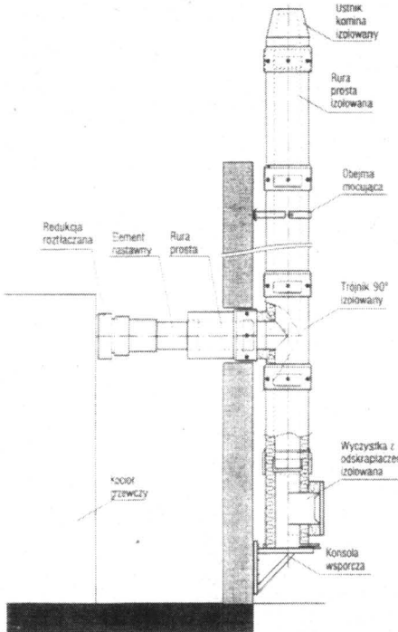
Części niezbędne do zbudowania kominu zewnętrznego
