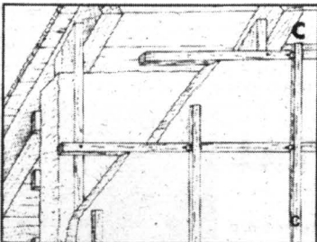
Mocowanie pionowych łatek montażowych albo kształtowników metalowych CD 60/27 w rozstawie maksimum 62,5 cm z zawieszami bezpośrednimi
