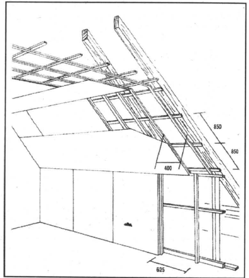
Przykładowa zabudowa: płyty ognioochronne 15,0 mm na łatach montażowych 50x30 mm (F30)
