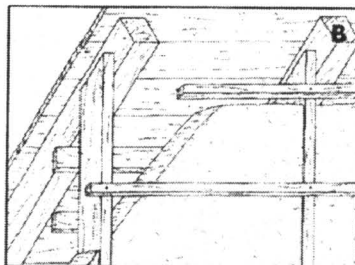
Zakładanie na dodatkowych warstwach izolacji poziomych łatek drewnianych
