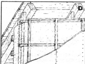
Okładanie płytami ognioochronnymi 15 mm. Krawędzie wzdłużnie płyt umieszcza się na pionowych łatach montażowych lub kształtownikach metalowych
