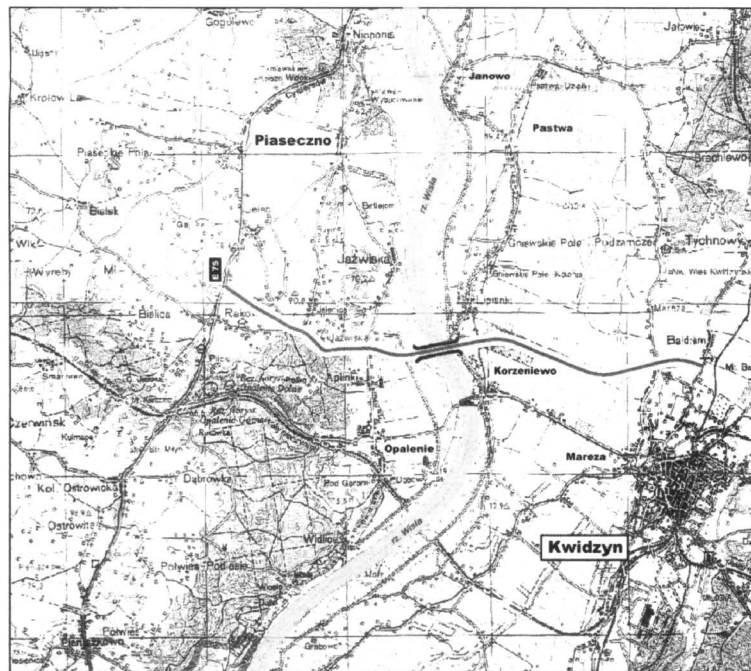
Orientacyjna mapa - budowa mostu przez Wisłę wraz z dojazdami
