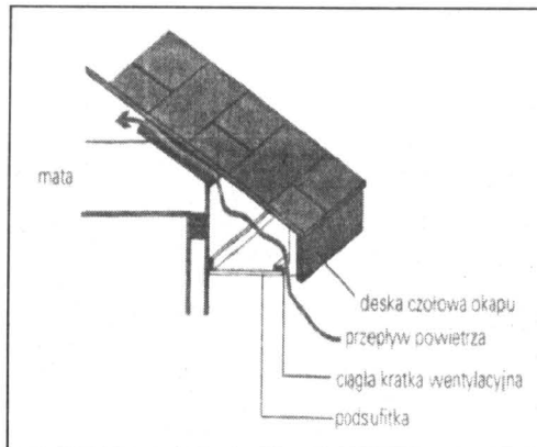
Okapowa wentylacja poddasza
