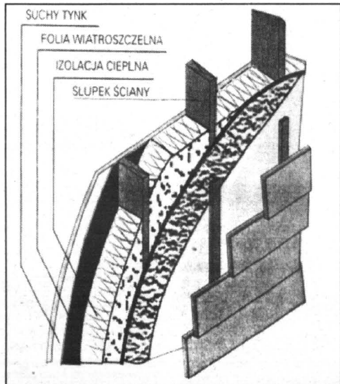
Układ warstw w ścianie budynku szkieletowego
