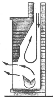
Brak półki dymowej powoduje, że gwałtowne uderzenia wiatru wypychają dym do pomieszczenia
