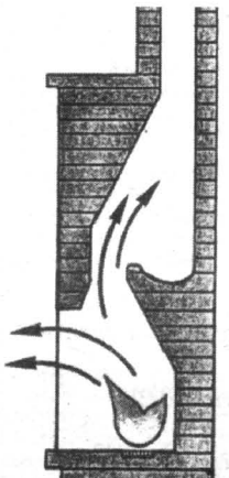
Półka umieszczona za nisko. Dym jest zbyt słabo zasysany do komina
