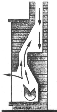
Niewłaściwie ukształtowana półka powoduje, że uderzenia wiatru tłumią ciąg kominka
