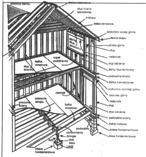
Rys. 1. Szkielet budynku wykonanego metodą platformową w technologii kanadyjskiej
