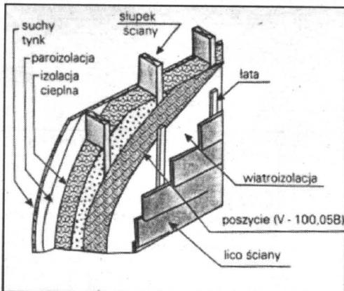
Rys. 6. Połączenie ściany zewnętrznej i wewnętrznej szkieletu
