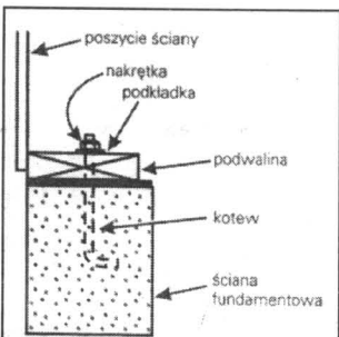
Rys. 2. Mocowanie podwaliny do fundamentów budynku
