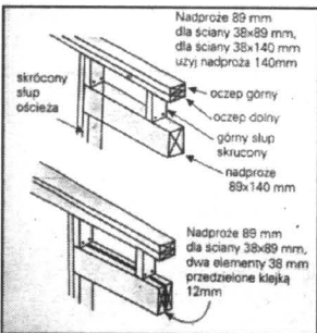
Rys. 4. Typowe rozwiązania nadproży okiennych
