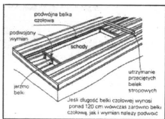
Rys. 3. Konstrukcja otworów stropowych
