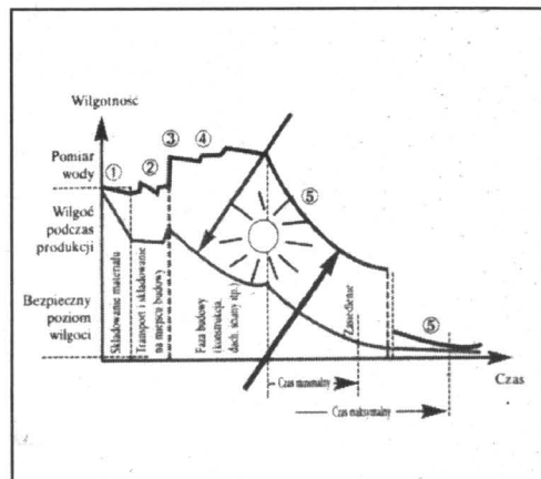
Rys. 2. Możliwości skrócenia czasu wykonywania prac budowlanych przy wykorzystaniu osuszania (w m3). Tylko techniczne osuszanie może wystarczająco zmniejszyć wilgotność w następujących sytuacjach: • Kiedy z powodu krótkich terminów naturalne schnięcie nie wystarcza. Dzięki osuszaniu rzemieślnicy, malarze, posadzkarze mogą wcześniej rozpocząć roboty. • Kiedy lokale położone są w piwnicach (kasy bankowe, magazyny). Przy utrudnionej cyrkulacji powietrza temperatura w pomieszczeniu jest niska. Przebieg zawilgoconia przy nieprzychylnych warunkach, gdzie techniczne osuszanie może przyspieszyć proces wykańczania pomieszczeń. 1. Niewłaściwe magazynowanie, np. brak zabezpieczenia przed deszczem; 2. Transport i magazynowanie materiału na budowie bez zabezpieczenia; 3. Zbyt duża ilość wody użyta do przygotowania zaprawy i betonu; 4. Pogoda i wiatr wpłynęły niekorzystnie na nie zamkniętą budowlę; 5. Z powodu czynników 1-4 utrzymuje się wysoka wilgotność. Akceptowany klimat wewnątrz budynku możliwy do osiągnięcia po nieproporcjonalnie długim czasie.
