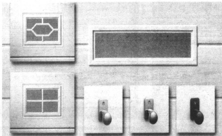
W bramach EcoTherm można zamontować estetyczne przeszklenia, a uchwyty do bram można wybrać wg indywidualnych upodobań z całej gamy okuć aluminiowych (w różnych kolorach) i stalowych
