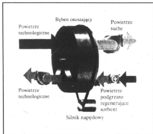
Rys. 1. Zasada działania bębna sorpcyjnego
