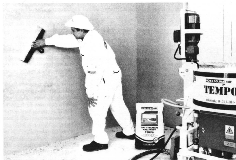
Wstępne, a później ostateczne wygładzanie powierzchni tynku gipsowego wykonuje się szpachlą długą, tzw. piórem
