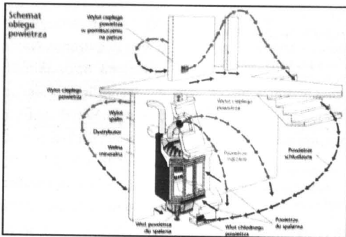
Schemat obiegu powietrza
