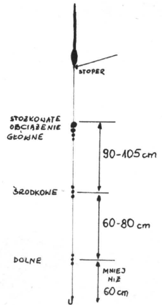
Rys. 2 Stożkowe obciążenie główne
